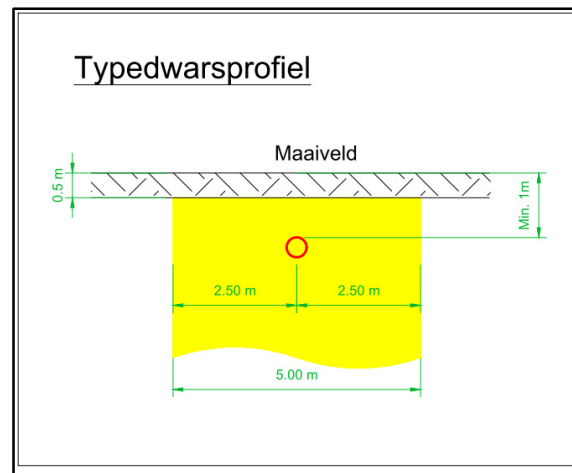
Dwarsprofiel ondergrondse inneming
