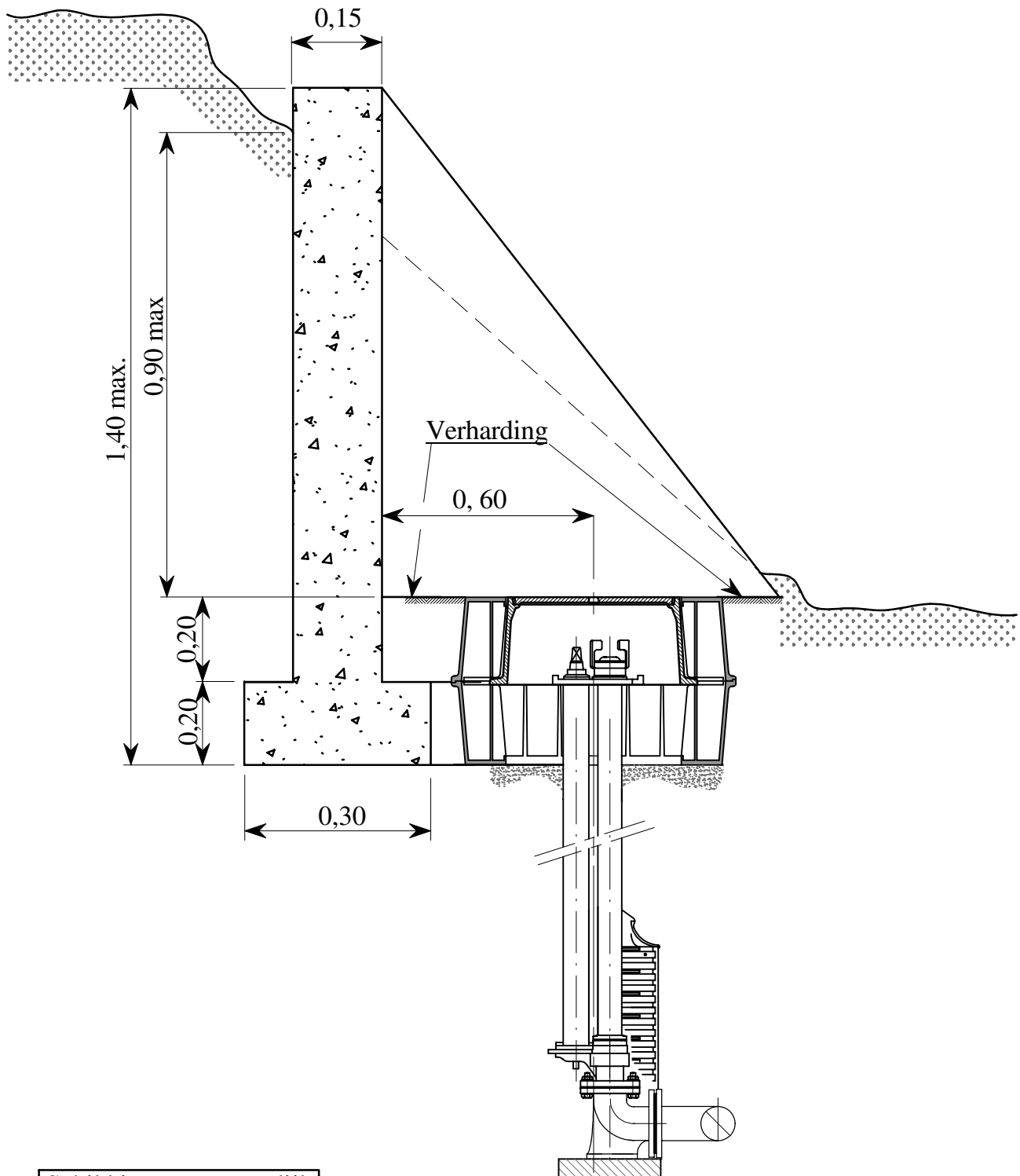
Doorsnede
